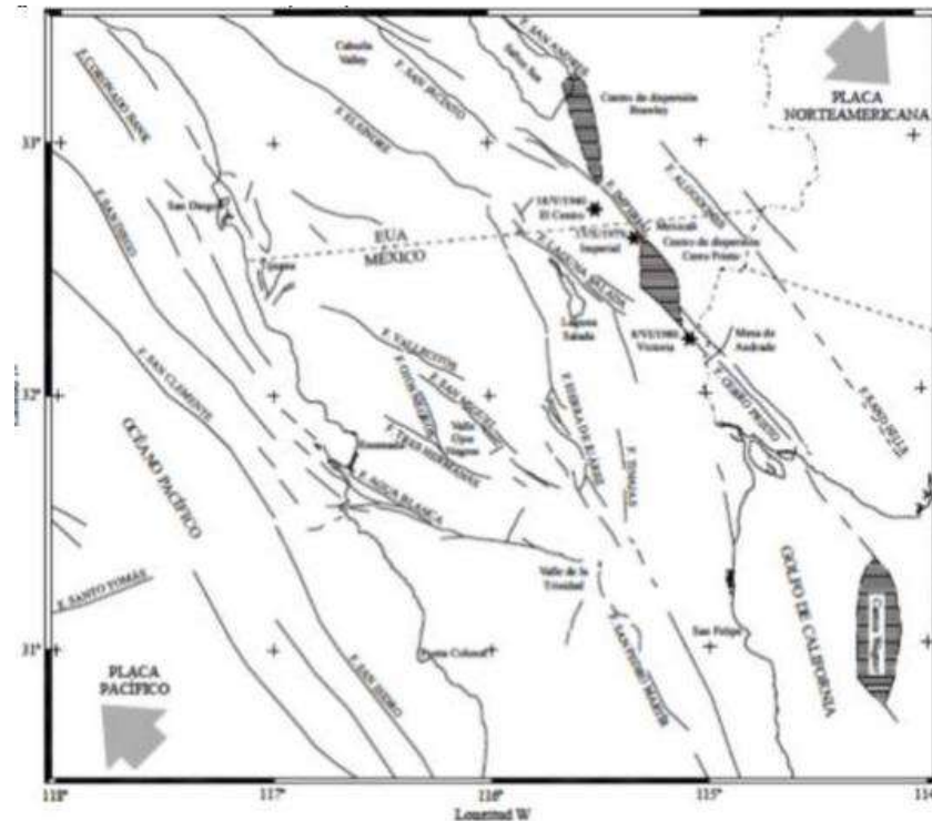
Figura 33. Distribución de las principales fallas activas asociadas al sistema de San Andrés-Golfo.
