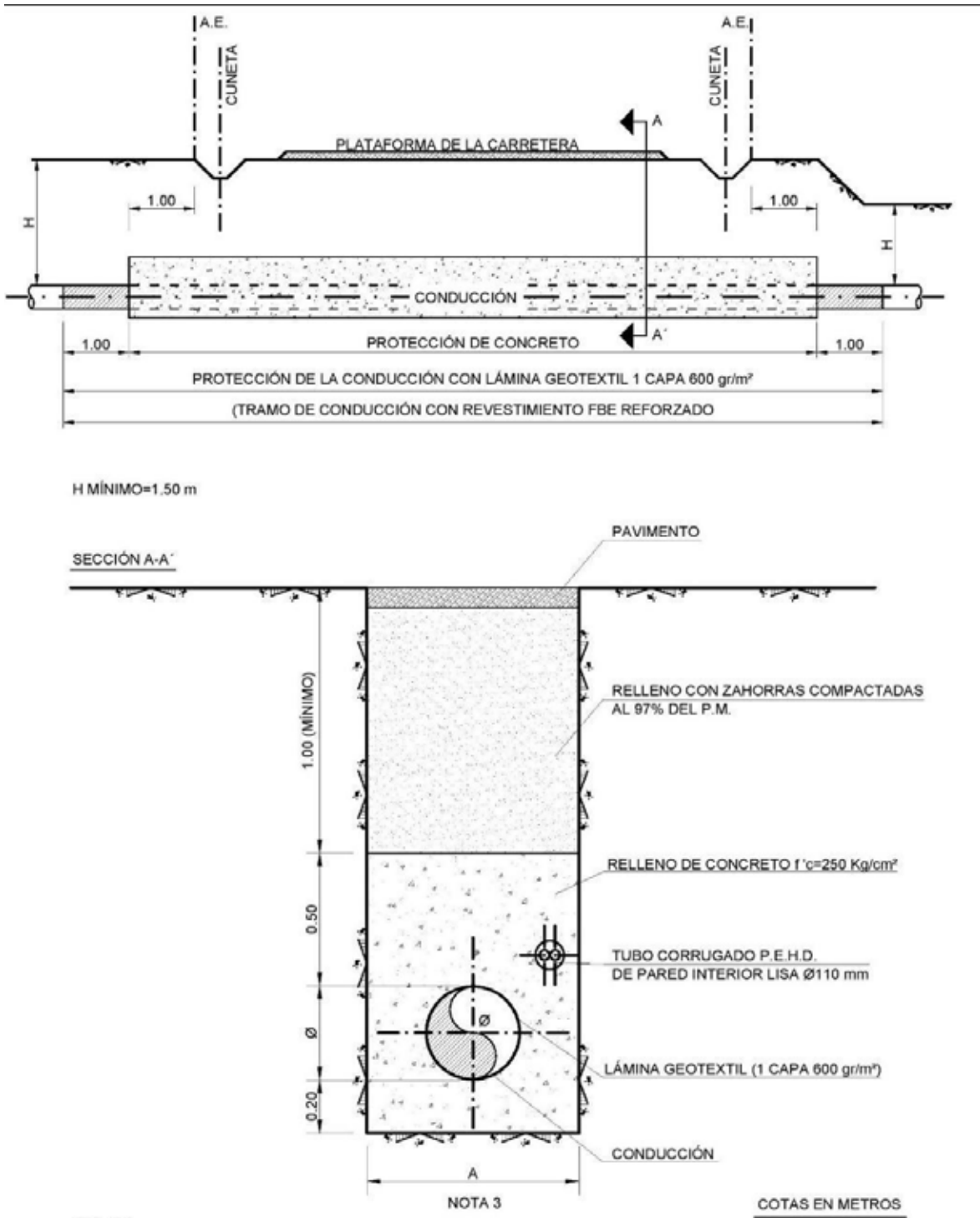
Figura 79. Cruce de carreteras a cielo abierto.
