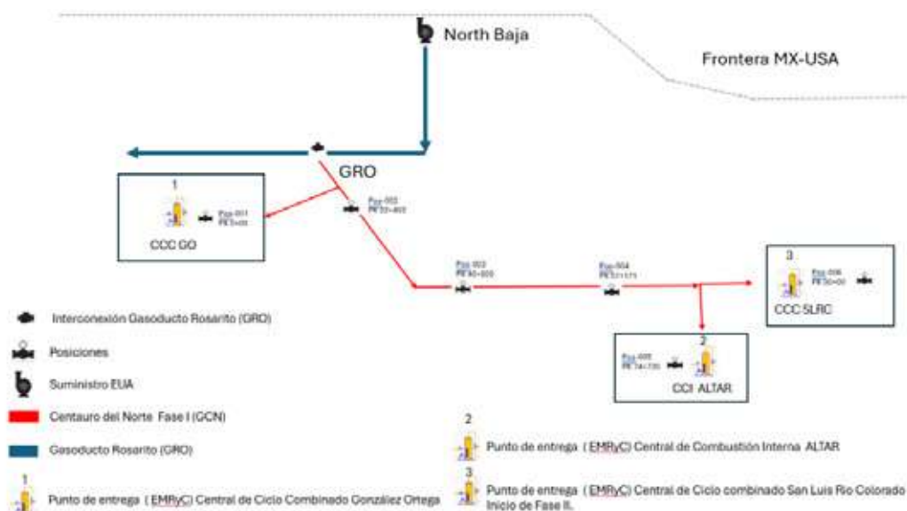
Figura 75. Esquema del Tramo I del Proyecto Gasoducto Centauro del Norte y su interconexión con el sistema existente Gasoducto Rosarito.
